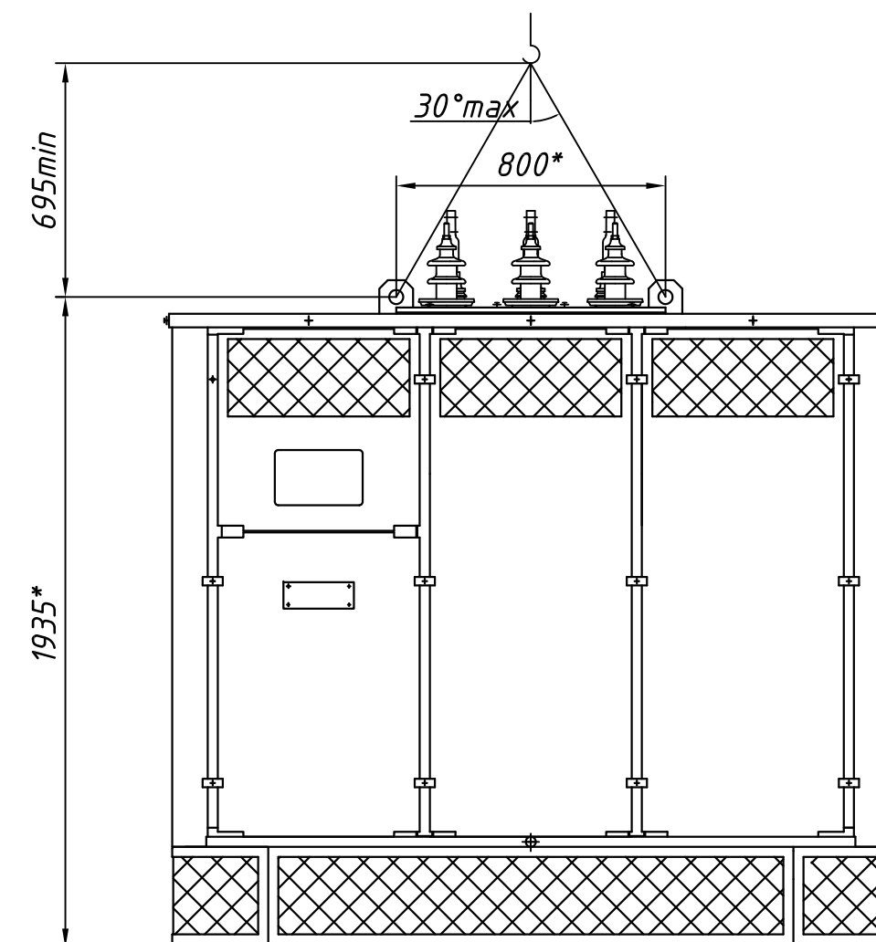
Схема подъема трансформатора
